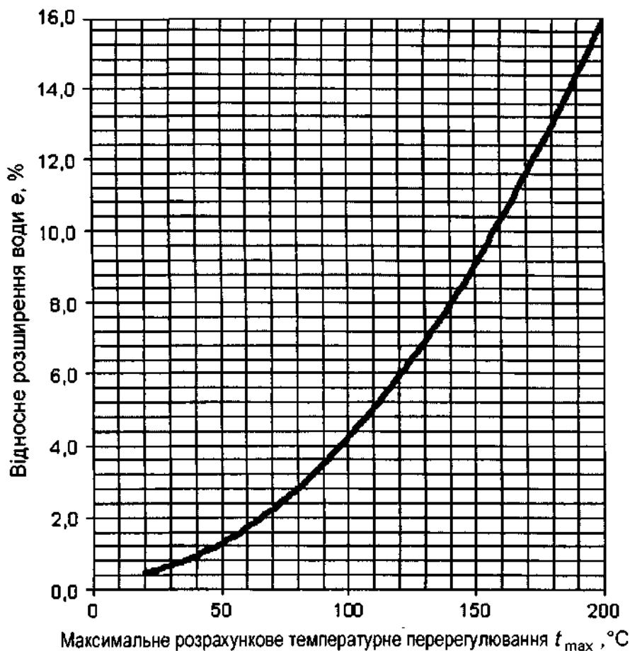
Рисунок Л.2 - Графічна залежність відносного розширення води від максимального розрахункового температурного перерегулювання за температури заповнення 10^\circ\text{C}
