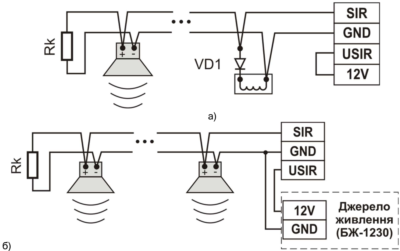
Рисунок 7.4 - Підключення оповішувачів:
