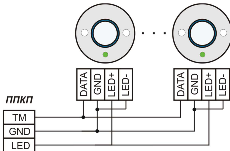
Рисунок 7.5 - Підключення Touch Memory
