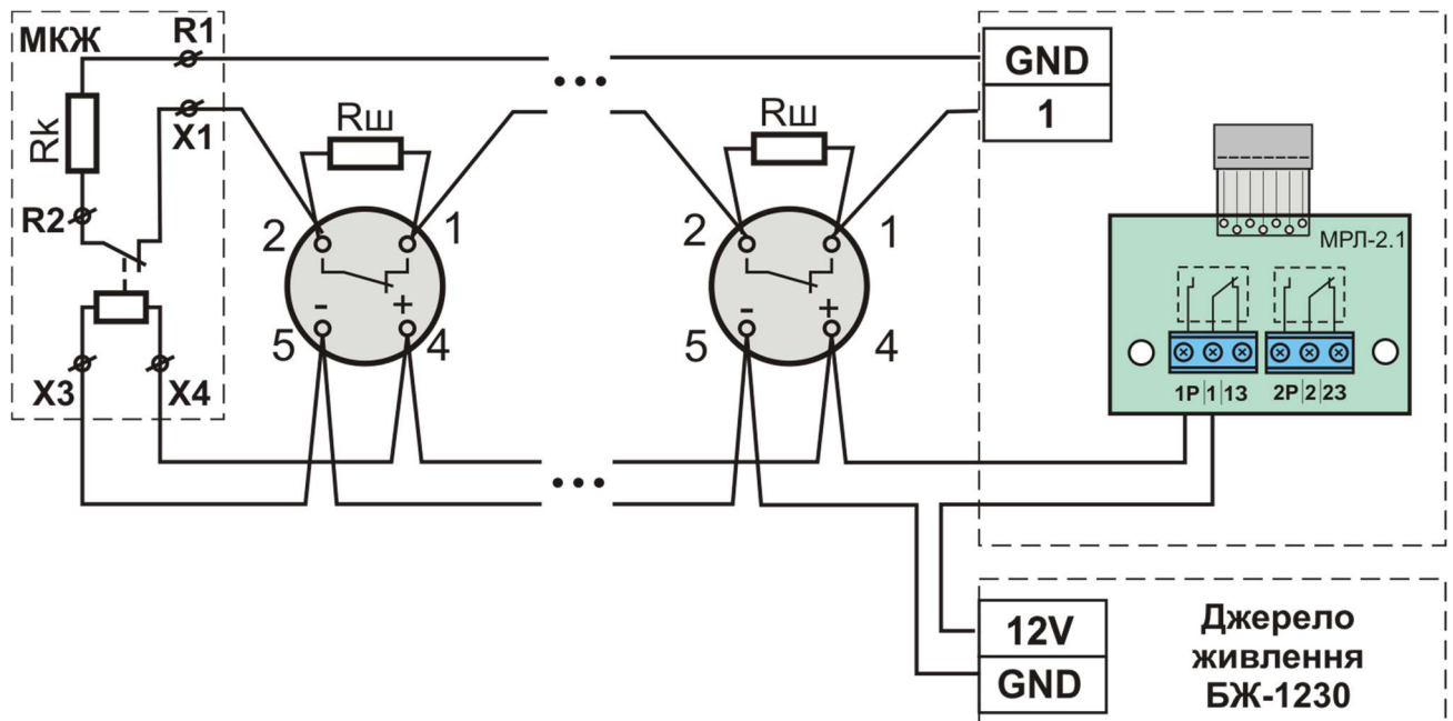
Рисунок 7.3 - Підключення чотиритровтових сповіщувачів з живленням від зовнішнього джерела живлення.
