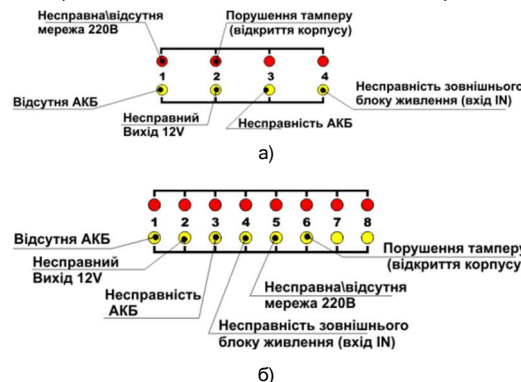
Рисунок 3 - Розширена індикація несправностей живлення: Тірас-4П (а), Тірас-8П (б)
