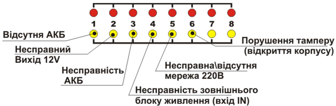
Рисунок 5.2 - Розширена індикація несправностей живлення для Тірас-8П
