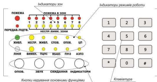
Рисунок 2 - Органи керування Тірас-8П.
