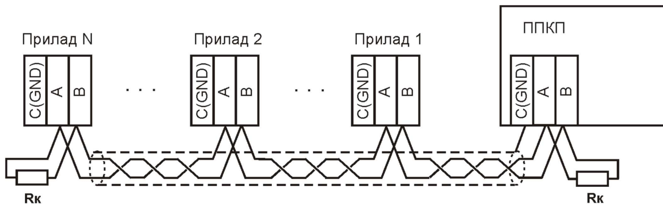
Рисунок 7.5 - Підключення інтерфейсу RS-485
