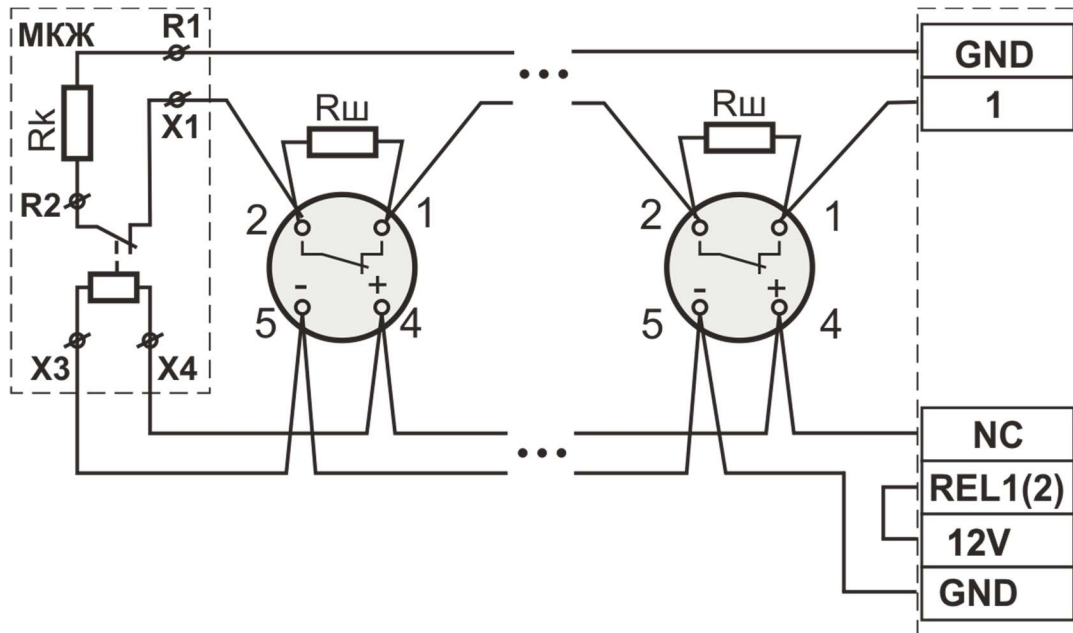
Рисунок 7.2 - Приклад підключення чотирипровідних сповісвачів з живленням від приладу.
