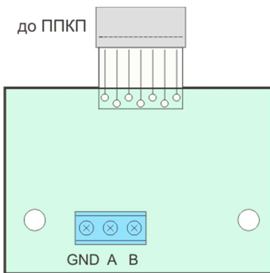
Рисунок 7.6 - Модуль МКІ
