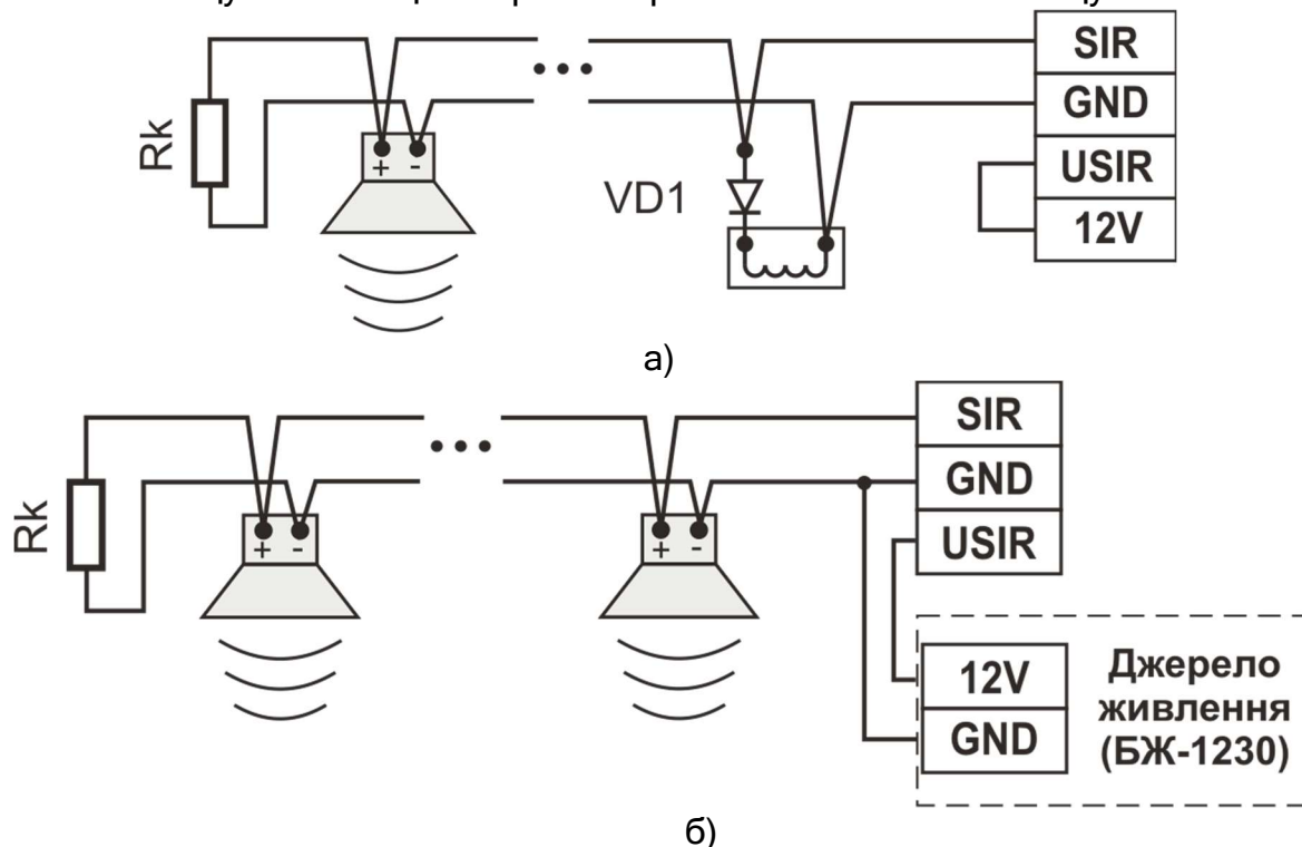
Рисунок 7.3 - Підключення оповісвачів: а) живлення від приладу, б) живлення від зовнішнього джерела живлення
