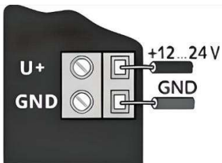
Рисунок 3 – Підключення провідників живлення панелі
