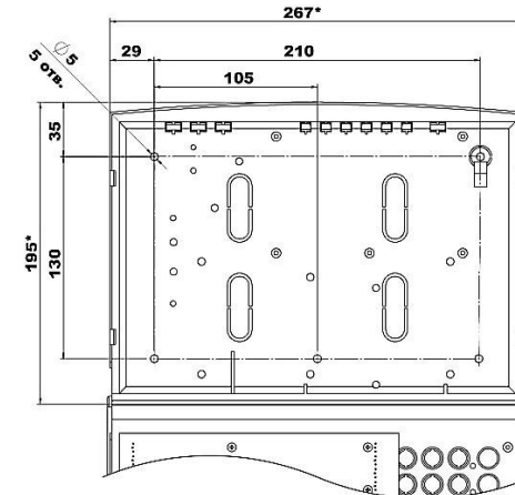
Рисунок 1- Розмітка отворів для кріплення панелі
