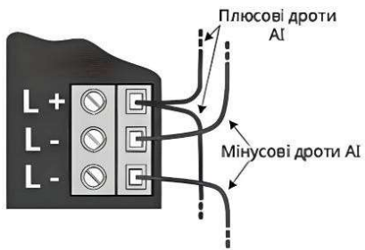
Рисунок 2 - Підключення провідників AI СПСА до клем AI панелі
