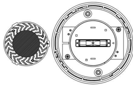
Рисунок 6.1 - Димова камера сповіщувача у відкритому стані
