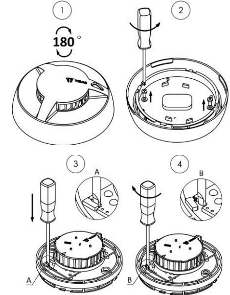
Рисунок 4.2 - Послідовність кроків для видалення ламкого елемента
