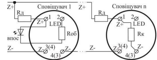
Рисунок 4.2 - Підключення ВПОС або світлодіода
