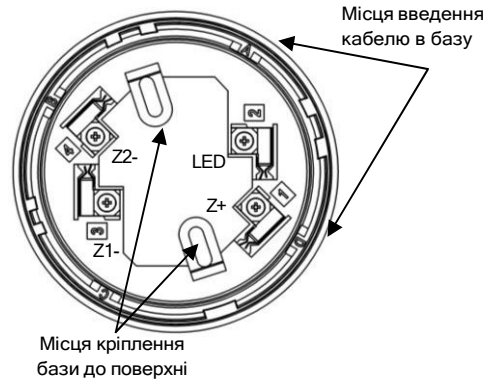
Рисунок 3.1 - Розташування клем на базі сповіщувача
