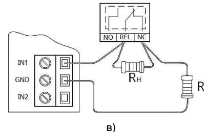
Рисунок 4.1 - Схеми підключень зовнішніх кіл до входів пристрою
