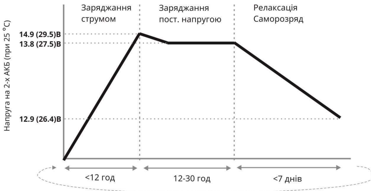
Рисунок 3.1 - Цикли роботи зарядного пристрою
