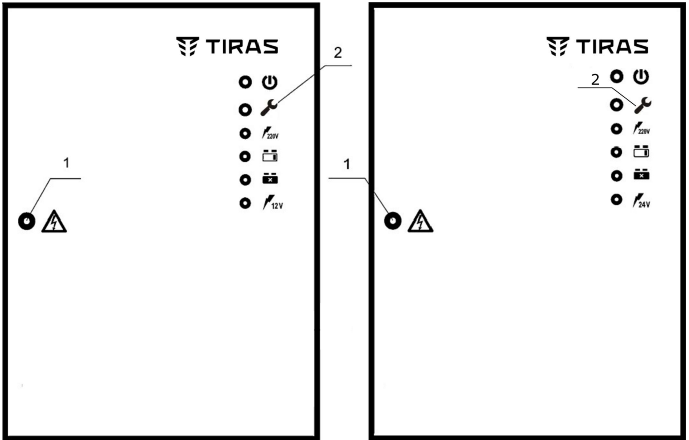
Рисунок А.1 - Зовнішній вигляд БЖ1230 (а) та БЖ2415 (б):
