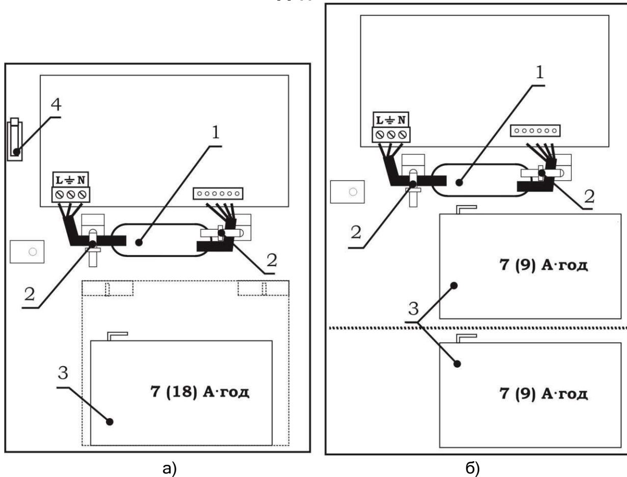
Рисунок В.1 - Компонівка БЖ1230 (а) та БЖ2415 (б):
