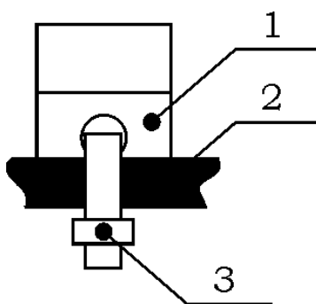
Рисунок В.2 - Спосіб кріплення проводів (Рис. В.1 поз. 2):
