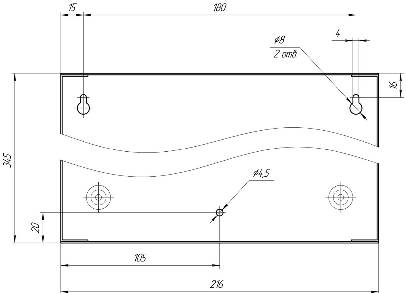
Рисунок Б.2 - Розмітка отворів для кріплення БЖ2415
