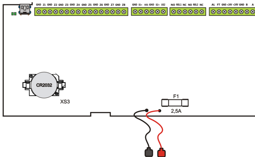
Рисунок 6 – Розміщення батареї годинника та запобіжника на основній платі
