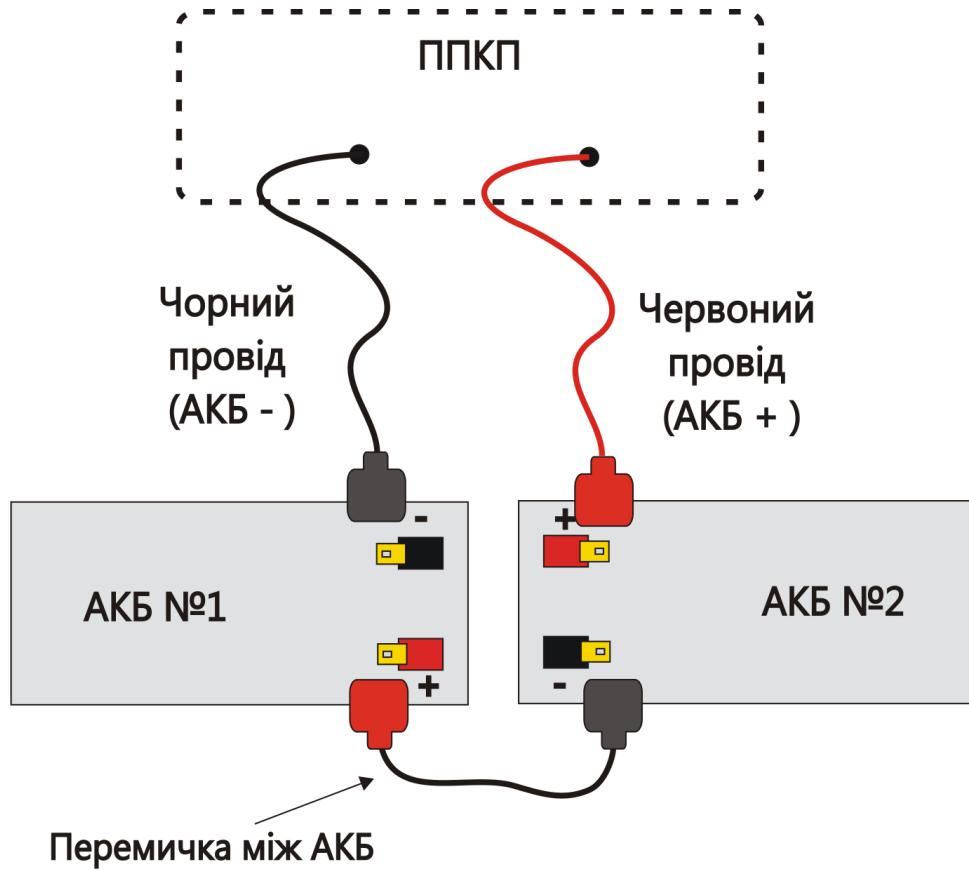
Рисунок 13 – Підключення АКБ
