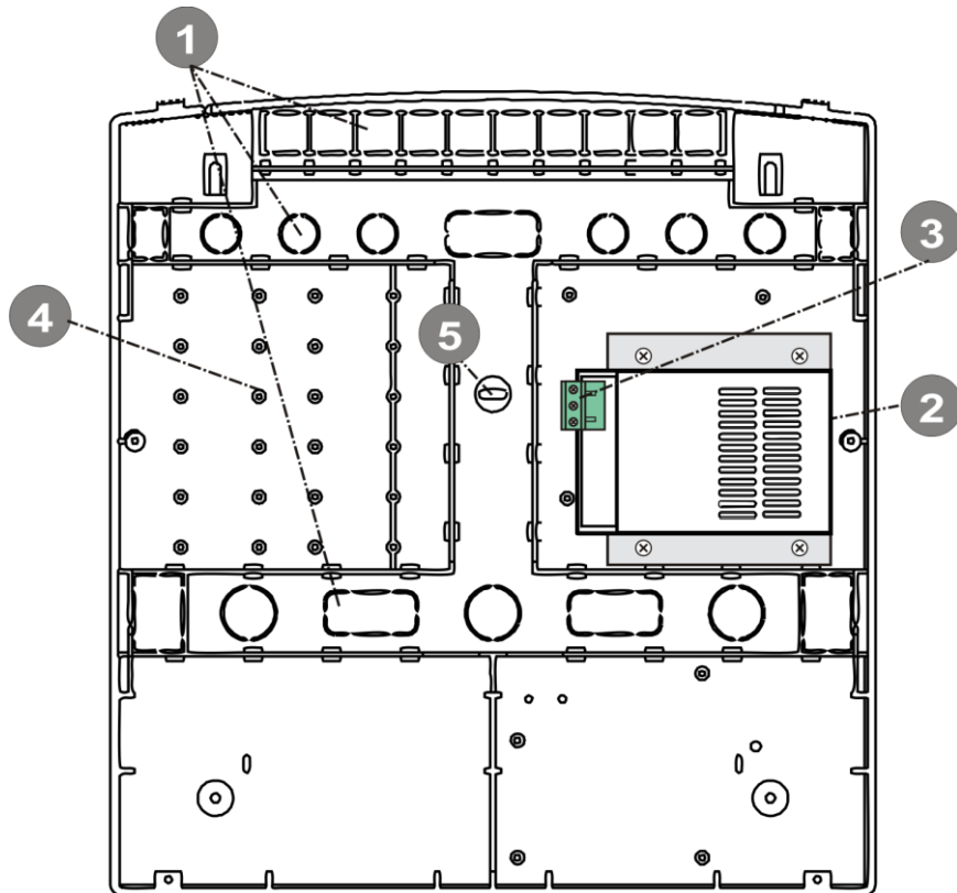
Рисунок 3 – Зовнішній вигляд корпусу без основного модуля «Tiras PRIME 8/16»:
