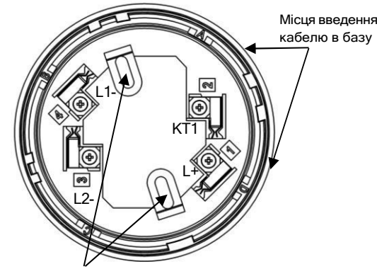
Рисунок 4.1 - Розташування клем на базі СПТА
