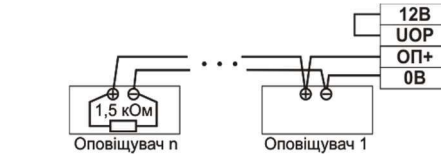
а) вихід оповіщення живиться від джерела живлення ППКП ПУІЗ;
