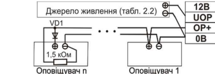
б) вихід оповіщення живиться від окремого джерела живлення.
