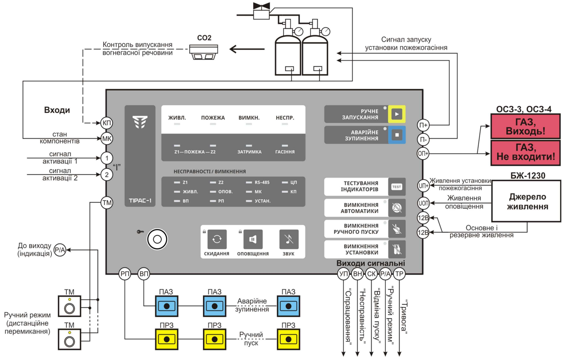
Рисунок А.6 - Приклад використання ПУЗ в системі газового пожежогасіння
