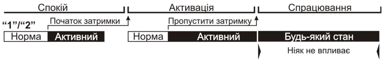
Рисунок 2.4 - Алгоритм роботи входів «1»/«2»
