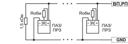
Рисунок А.3 - Підключення ПР3 та ПА3 до входів «РП» та «ВП» за двопровідною схемою (додаткові відомості з підключення - див. паспорт на ПА3 або ПР3)
