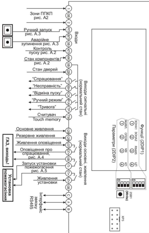
Рисунок А.1 - Підключення входів та виходів
