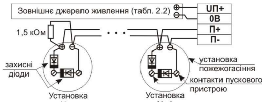
Рисунок А.5 - Підключення до пускових пристроїв установки пожежогашіння.
