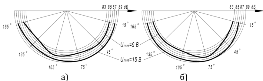
Рисунок 1 – Акустичні діаграми оповіщувача: а) – робоча позиція, б) – розвернута на 90° за годинниковою стрілкою позиція.
