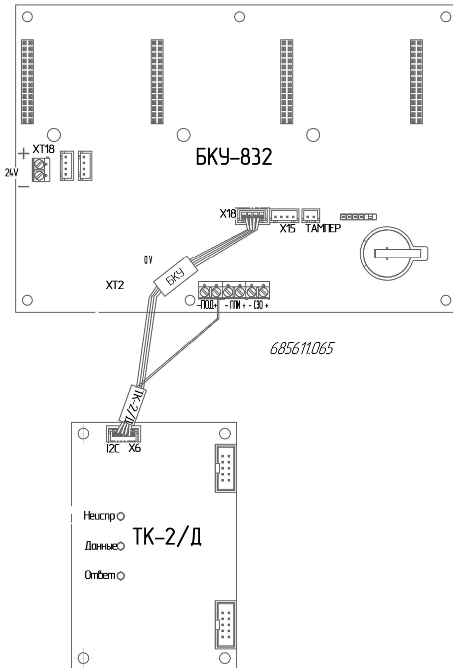
Схема подключения ТК-2/Д к БКУ-832
