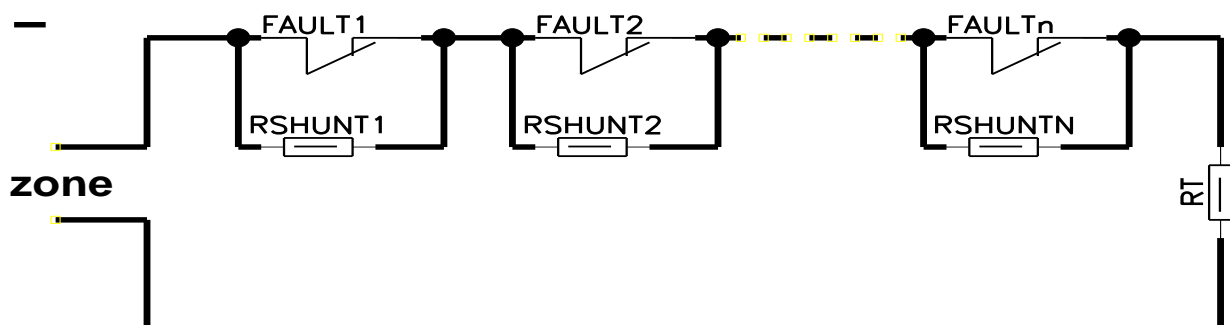
Малюнок 6 – Підключення контактів «FAULT» до шлейфу сигналізації по схемі АБО (OR) з визначенням обриву шлейфу
