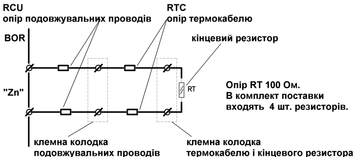
Малюнок 1 – Схема підключення термокабелю
