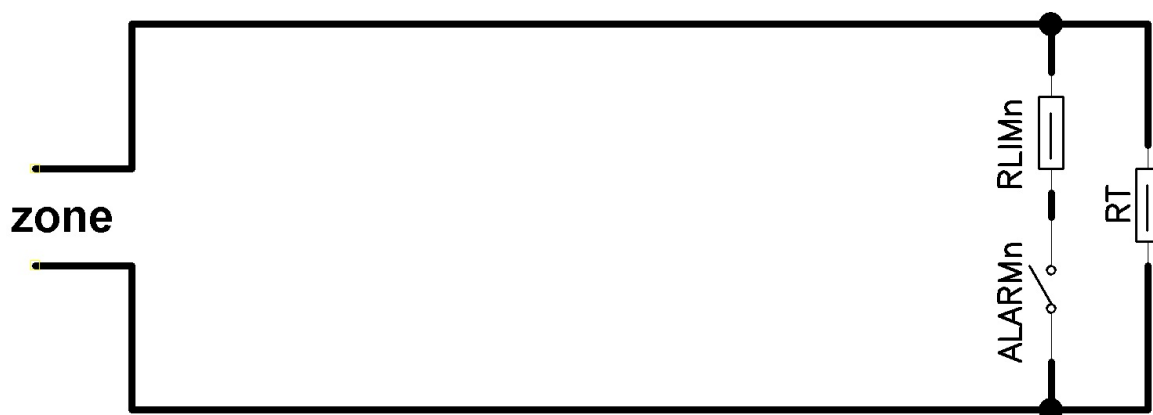
Малюнок 2 – Підключення поодиноких контактів «ALARM» блоку до шлейфів сигналізації
