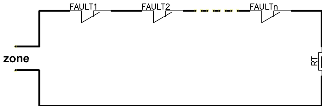
Малюнок 5 – Підключення контактів «FAULT» блоку до шлейфу сигналізації по схемі АБО (OR)
