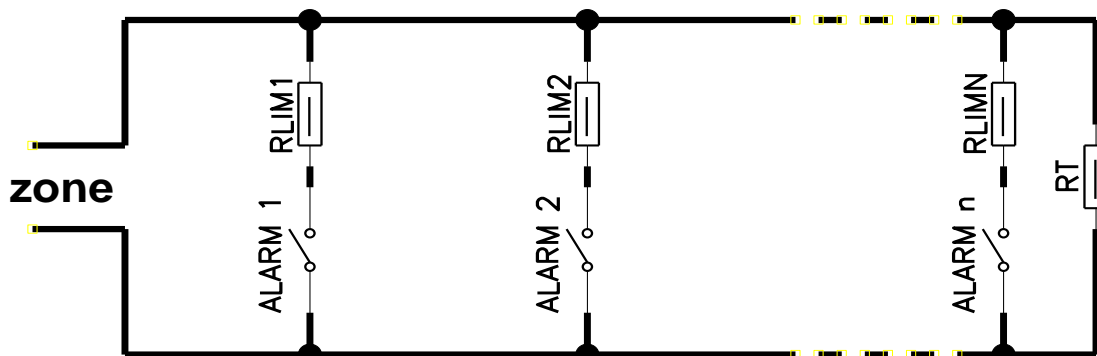
Малюнок 3 – Підключення контактів «ALARM» блоку до шлейфу сигналізації по схемі АБО (OR)
