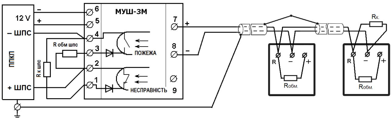
Рис. 6 Схема підключення сповісвачів до чотирипровідного знакозмінного ШПС за допомогою модуля МУШ-3М
