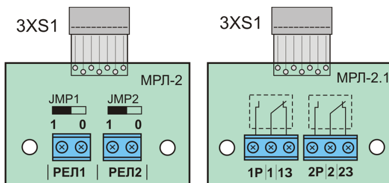
Рисунок 7.9 – Модулі МРЛ
