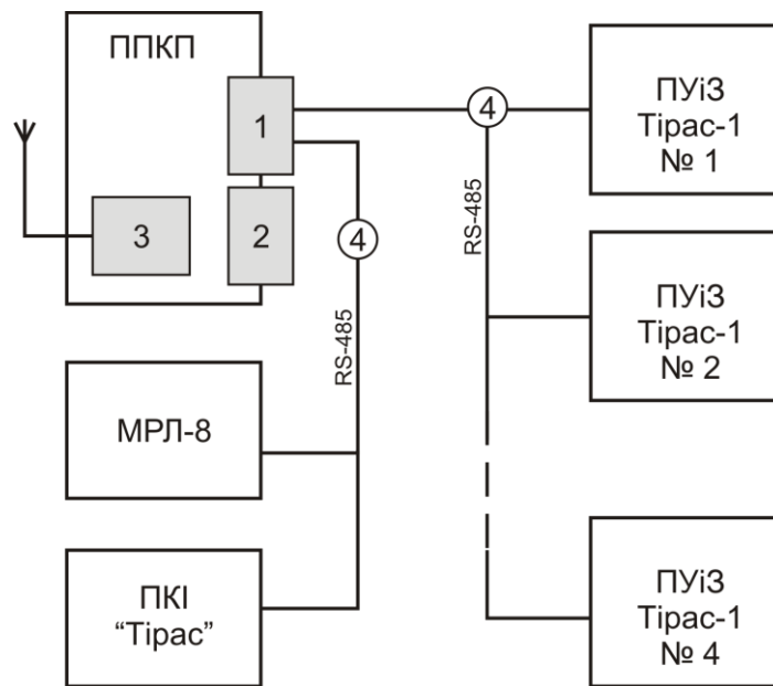
Рисунок 3.1 – Приклад СПС:
