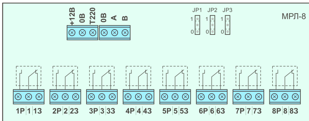
Рисунок 7.10 – Підключення входів та виходів МРЛ-8
