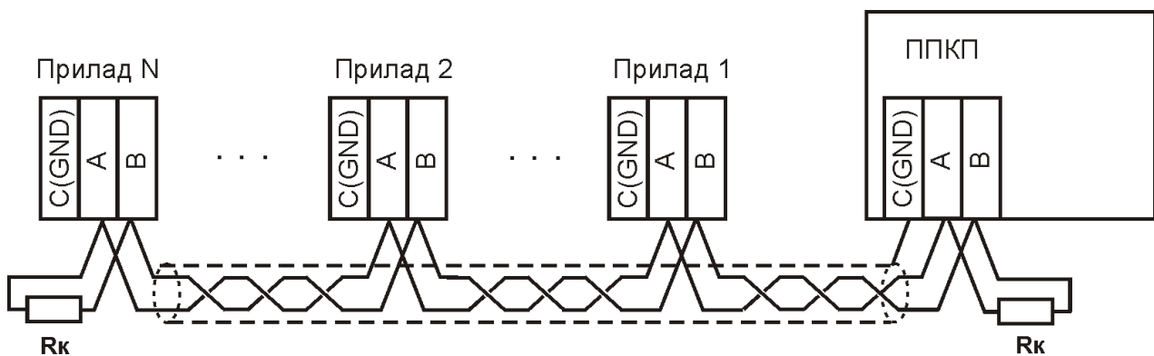
Рисунки 7.6- Підключення інтерфейсу RS-485 без відгалужень
