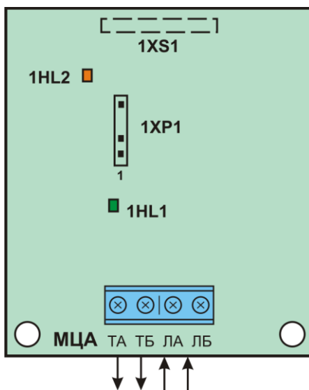
Рисунок 7.11 – Підключення входів та виходів МЦА
