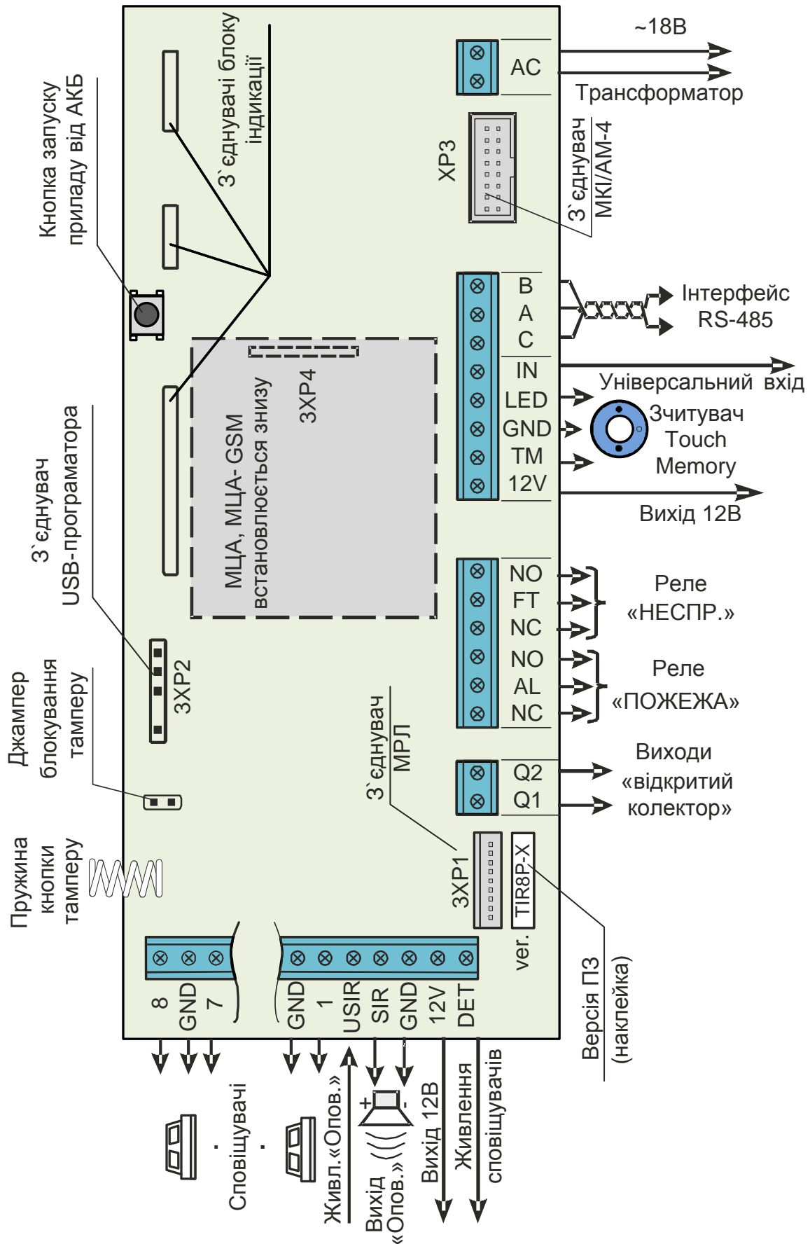
Рисунок Г.1 – З'єднання ППКП
